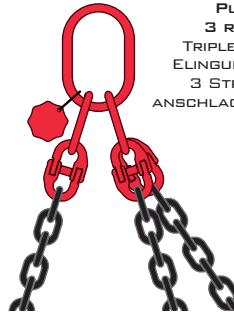
PULPO DE 2 RAMALES DOUBLE SLINGS ÉLINGUE DOUBLE 2 STRÄNGIGE ANSCHLAGKETTEN
